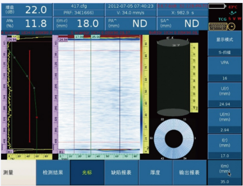
无裂纹螺栓检测图像
